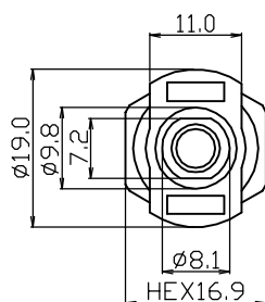
PSW-A4F外観図
