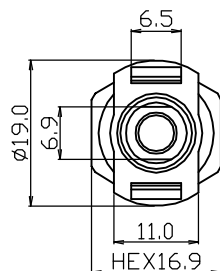
PSW-A4F外観図
